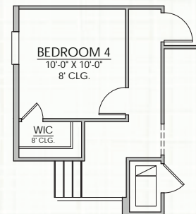
Optional Bedroom 4 In Lieu of Loft
